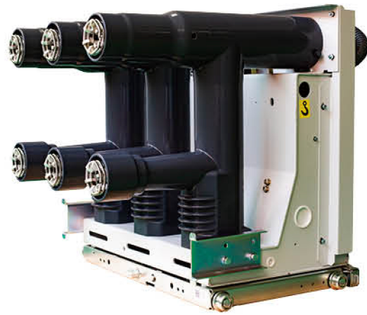
新一代 SCL(R)-12 移开式真空负荷开关 - 熔断器组合电器
